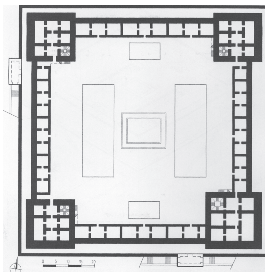
איור 10: הקומה השנייה באנטוניה לפי נצר. מתוך: נצר תשס"ח.
